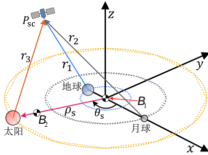
图2 BCR4BP (E-M 旋转系)
