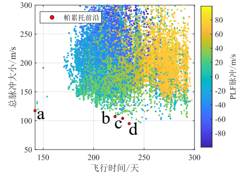
图13 全局修正解空间 Fig.13 Global correction of solution space
