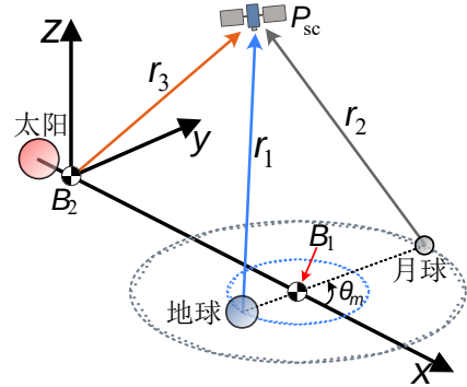
图3 BCR4BP (S-B1 旋转系)
