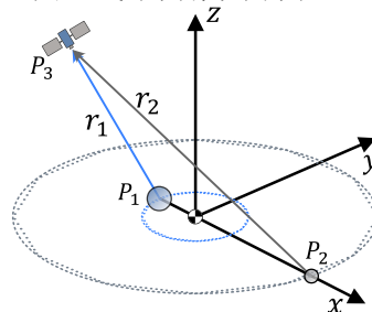
图1 CR3BP 示意图
