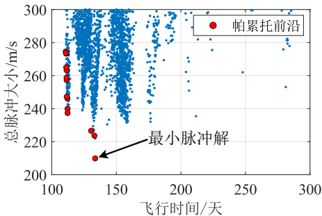
图22 直接转移解空间 Fig.22 Direct transfer solution space
